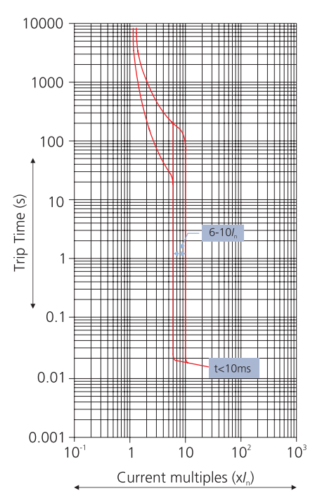
DN3 MCCB
